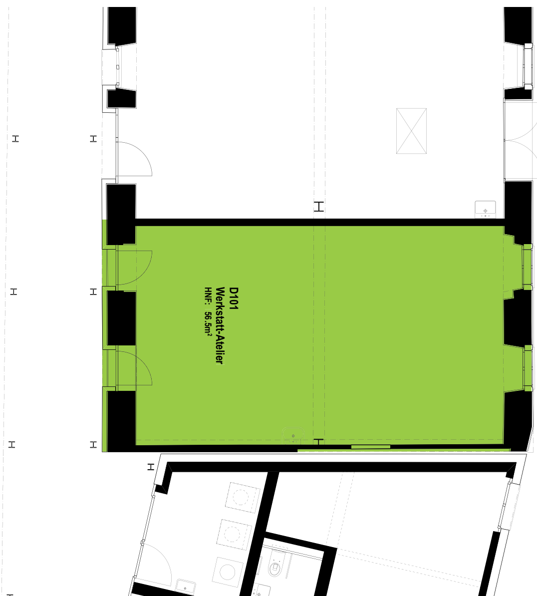
Grundriss 1:100
