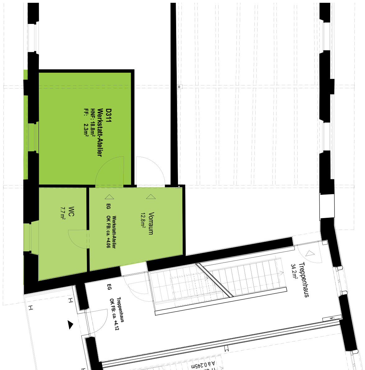
Grundriss 1:100
