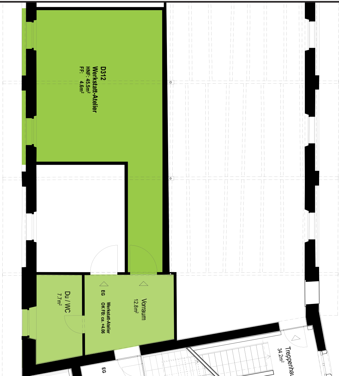
Grundriss 1:100
